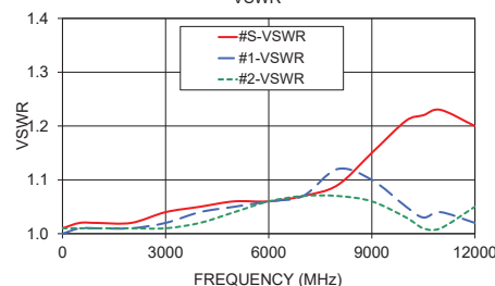
ZFRSC-123-S+ VSWR
