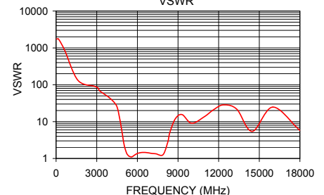
VBFZ-6260+ VSWR
