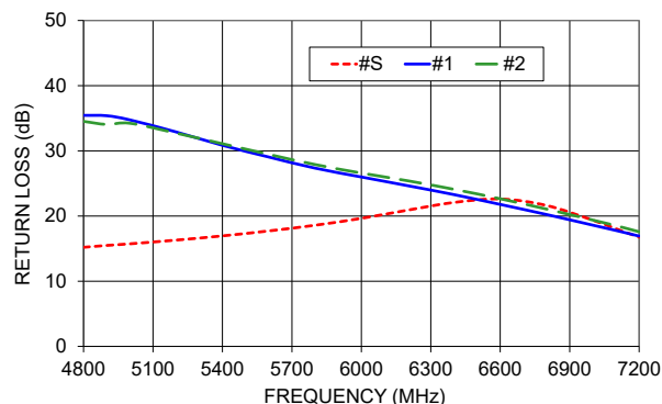
SCW-2-722+ RETURN LOSS
