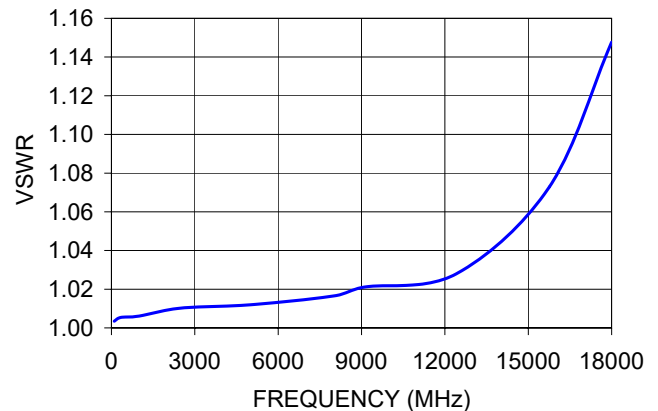
BW-S5W2+ VSWR
