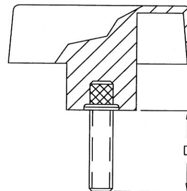
THREADED STUD
