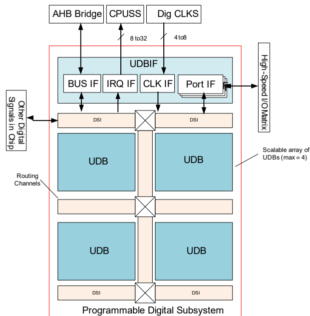
Figure 5. UDB Array
