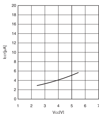
I_{CCTS} - V_{CC}
