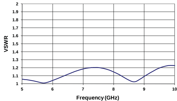
VSWR (5-10 GHz)
