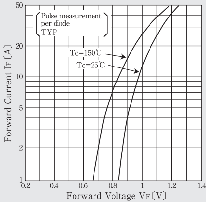
順方向特性 Forward Voltage
