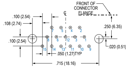
15 SOCKET MWDM-15SCBR
