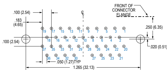
37 SOCKET MWDM-37SCBR
