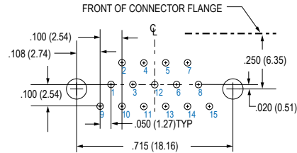
15 PIN MWDM-15PCBR
