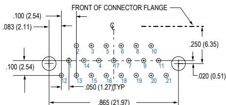
21 PIN MWDM-21PCBR
