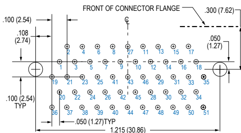
51 PIN MWDM-51PCBR
