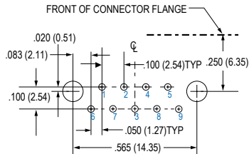
9 PIN MWDM-9PCBR
