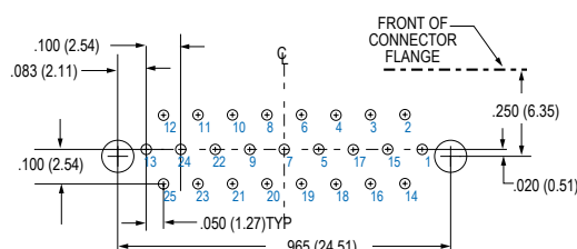
25 SOCKET MWDM-25SCBR
