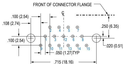
15 PIN MWDM-15PCBR
