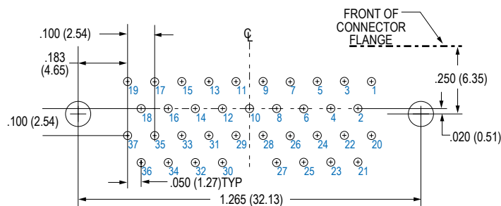
37 SOCKET MWDM-37SCBR
