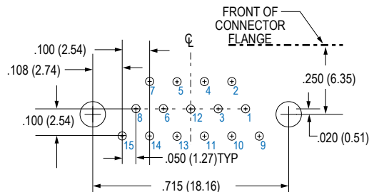
15 SOCKET MWDM-15SCBR
