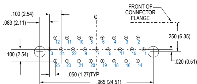
25 SOCKET MWDM-25SCBR
