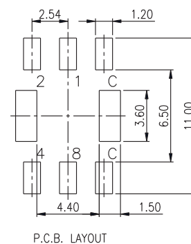
P.C.B. LAYOUT
