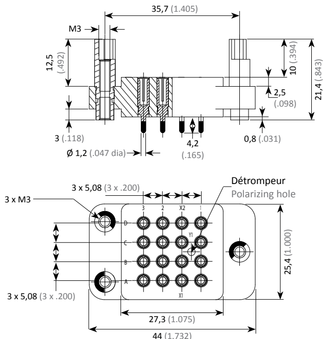
Dimensions avec colonnettes détrompées Dimensions with polarized pillars
