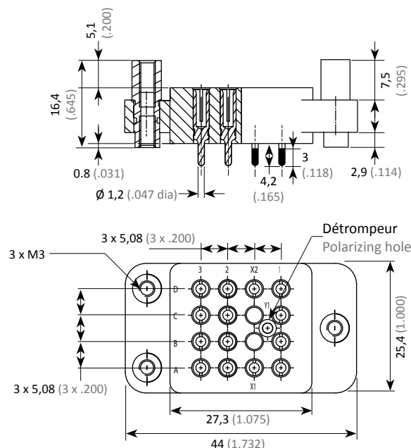
Dimensions avec colonnettes non détrompées Dimensions with not polarized pillars
