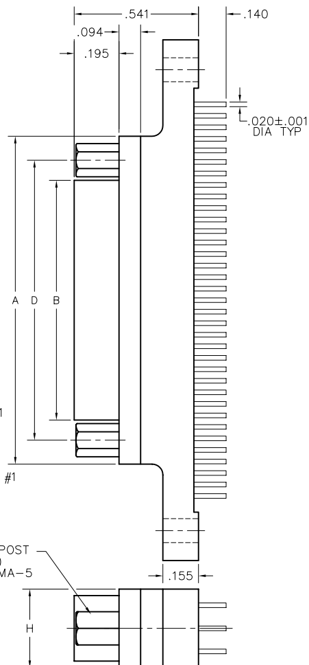
RECEPTACLE
