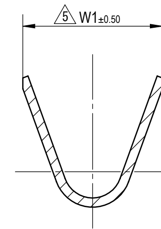
SECTION A-A
