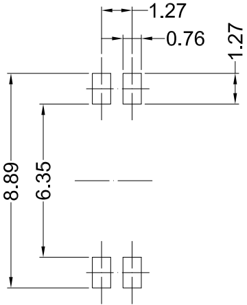
P.B.C LAYOUT
