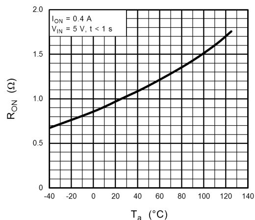
Fig. 12.4 R_{ON} - T_a
