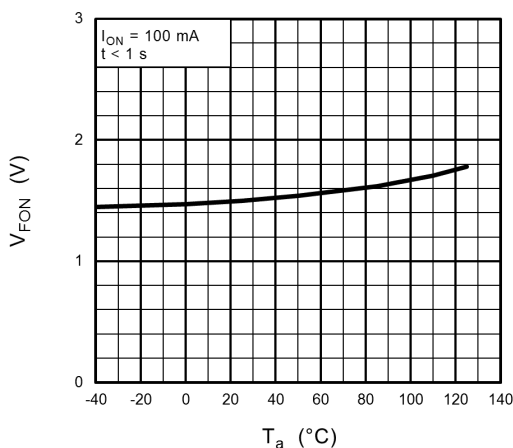
Fig. 12.5 V_{FON} - T_a
