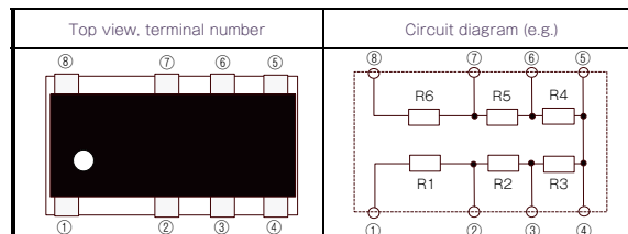
RM11264(11.2mm×6.4mm)
