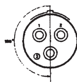
23 3 contacts \varnothing 2,5 mm
