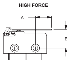
FIG. 3 Lever
