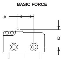
FIG. 7 Pin Plunger
