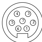
7 Pole
