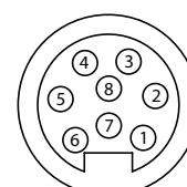
8 Pole
