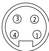
4 Pole
