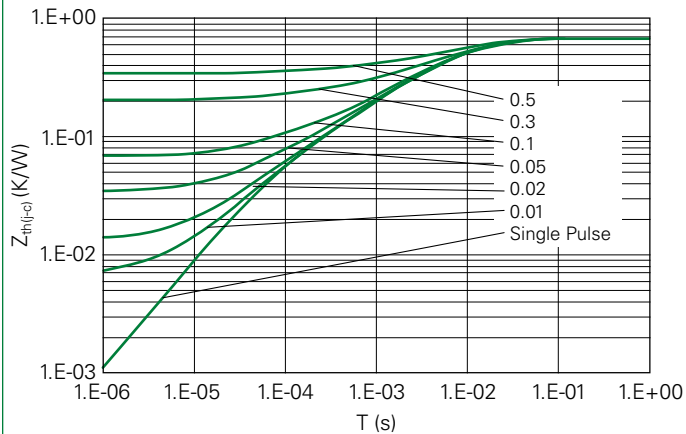
Fig. 7. Transient Thermal Impedance
