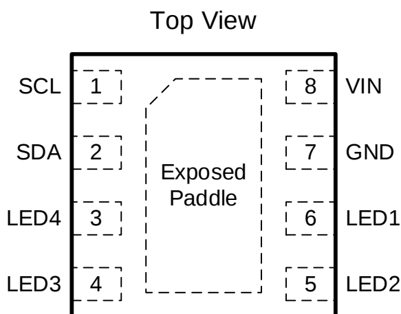
UDFN22-8
