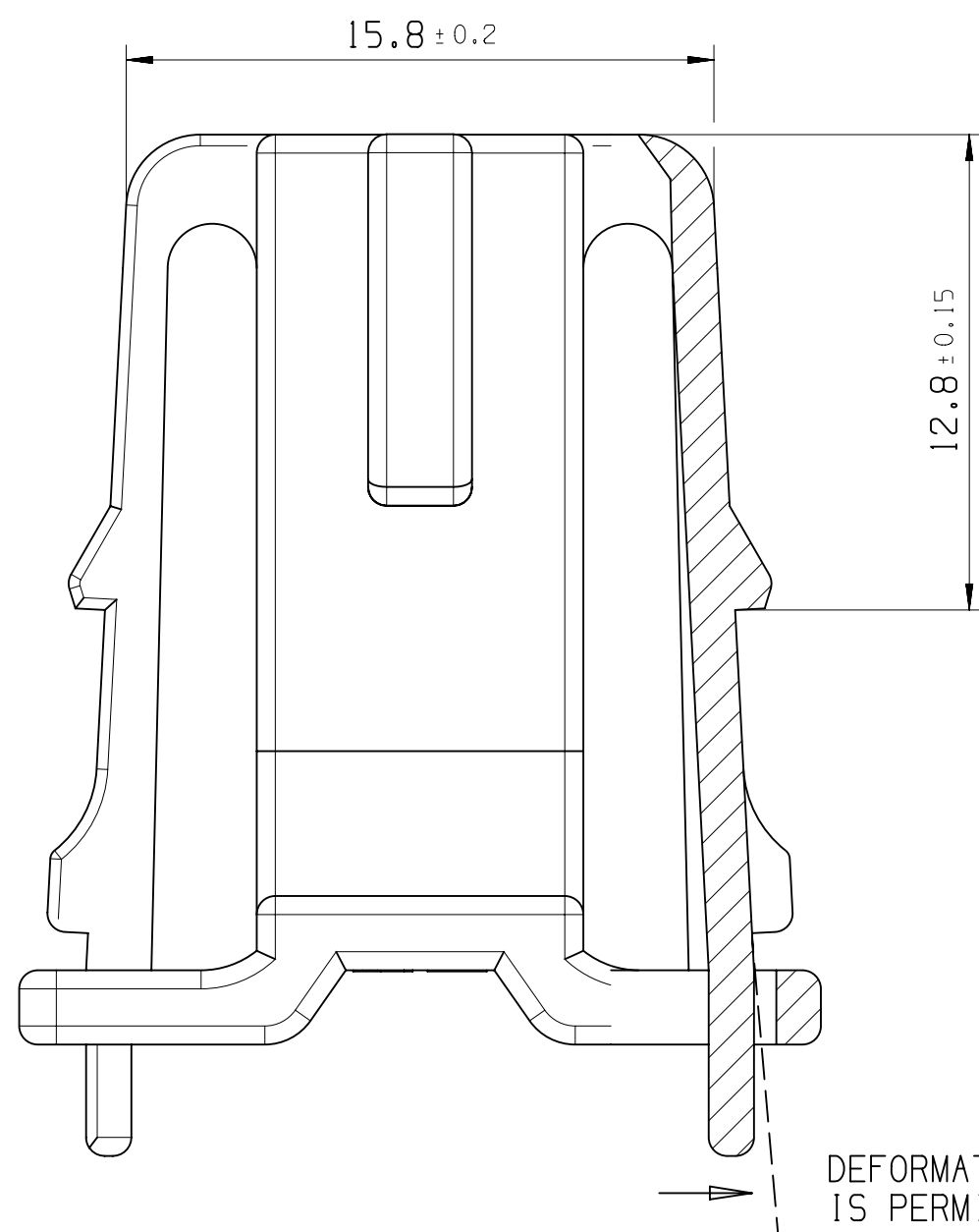
SECTION A-A 5:1
