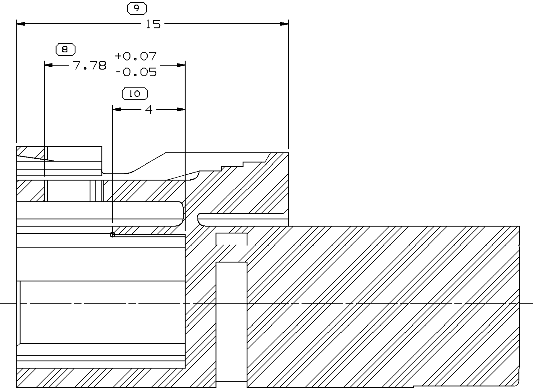
SECTION A-A
