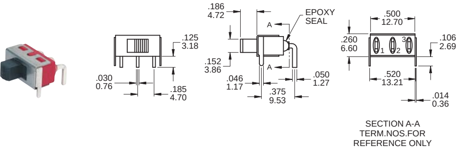
SPDT
