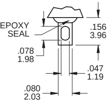
M1 Solder lug
