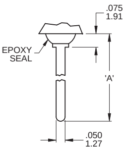
M5 Wire Wrap
