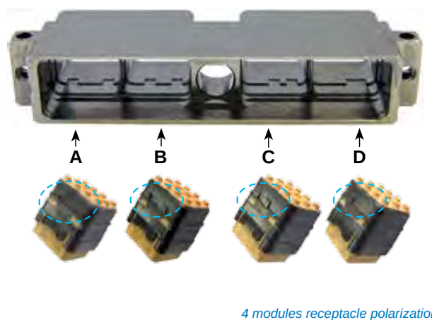
Polarisation d'une embase 4 modules
