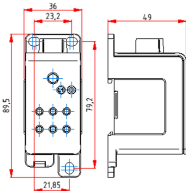
Montagehinweise | Assembly Details | Montage
