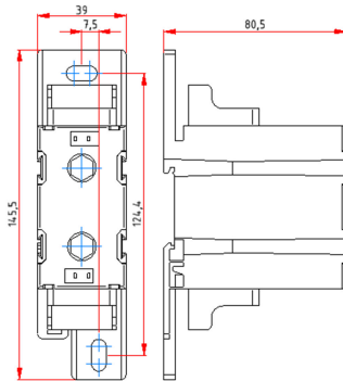
Maßzeichnung | Dimensional Drawing Plan d'encombrement
