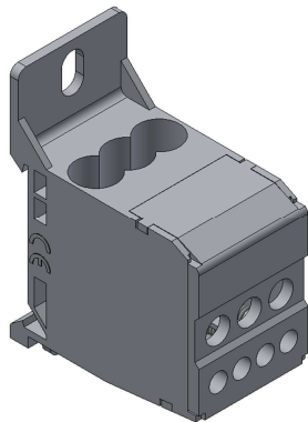
Maßzeichnung | Dimensional Drawing Plan d'encombrement
