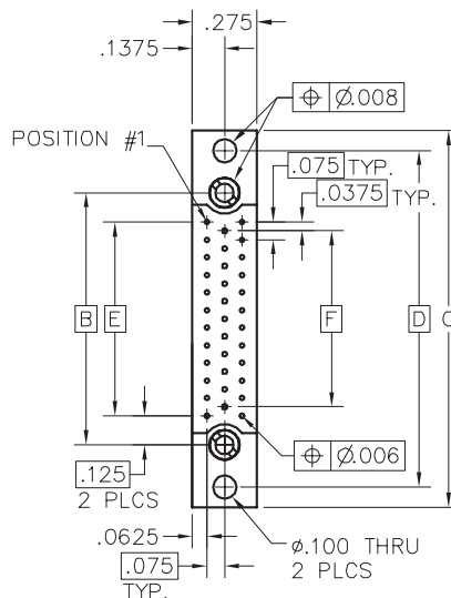
RECEPTACLE
