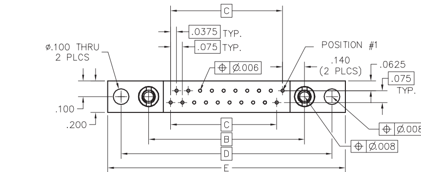
RECEPTACLE
