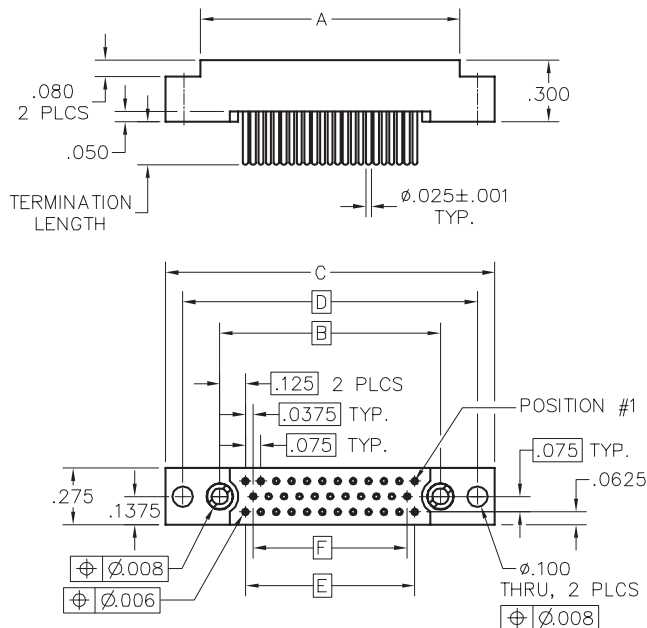
RECEPTACLE
