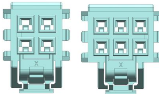
4ckt & 6ckt Receptacle
