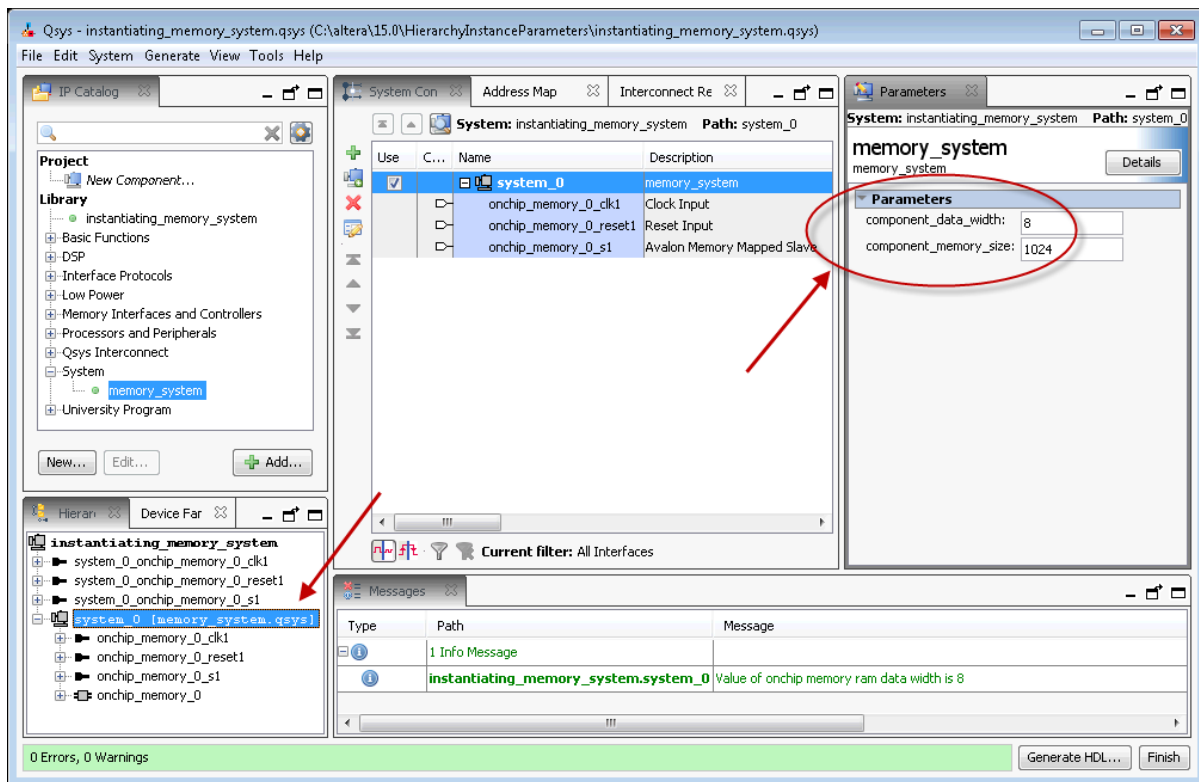
Figure 5-22: Displays memory_system.qsys Instance Parameters in the Parameter Editor
