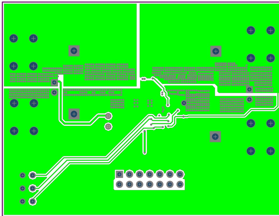
Copper Layer 3
