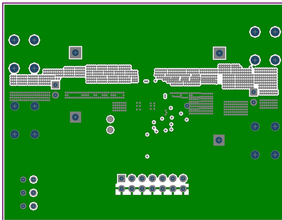
Copper Layer 2
