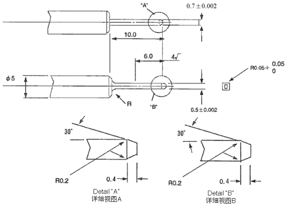
图表 8 端子插拔力测试用量规规格
