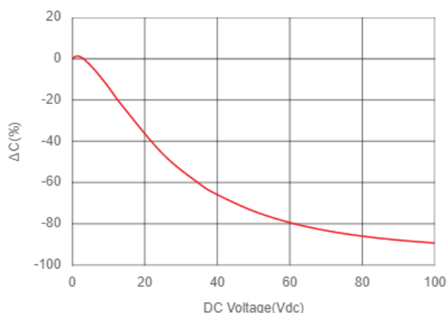
Figure5. CL32Y106KCVZNWE DC-Bias
