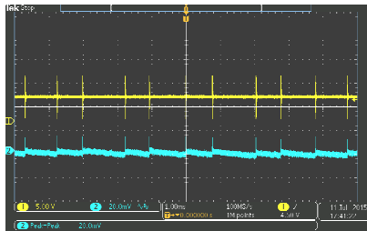
Vin=10V Vout=5V Iout=0A
