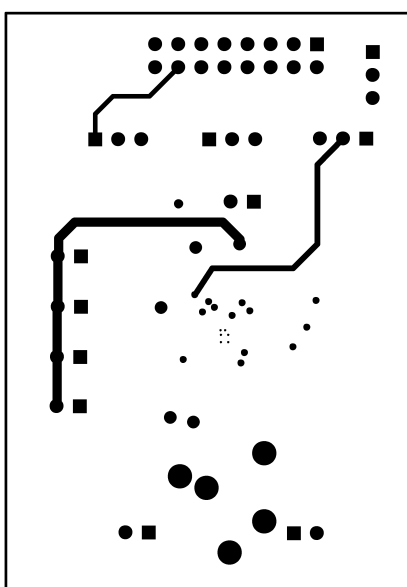
Figure 45. Bottom Layer
