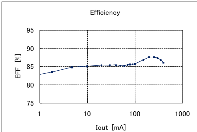
Vin=5.0V, Vout=3.0V
