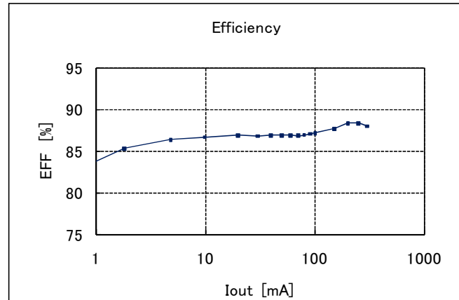
Vin=5.0V, Vout=3.3V
