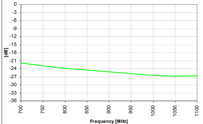
CMRR
