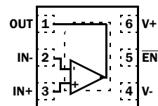
ISL28191
