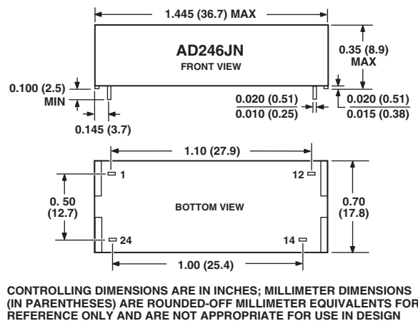
AD246JN Package
