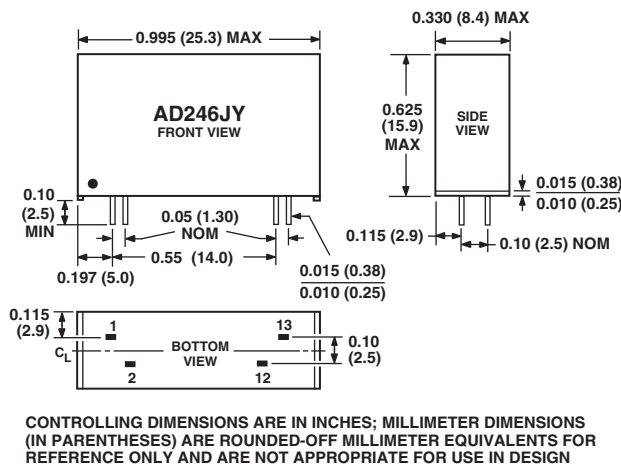
AD246JY Package
