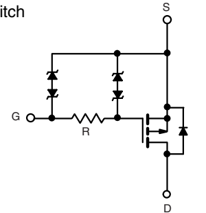
P-Channel MOSFET
