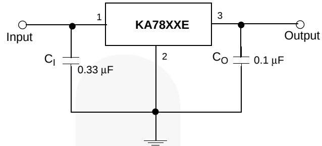
Figure 6. DC Parameters
