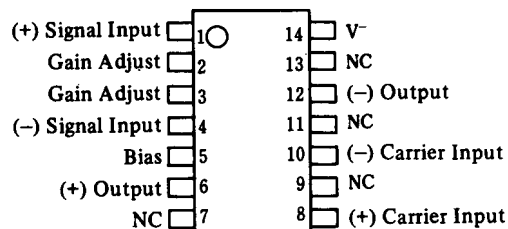
NJM1496D NJM1496M NJM1496V
