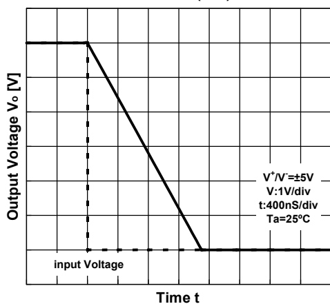
Slew Rate(Fall)
