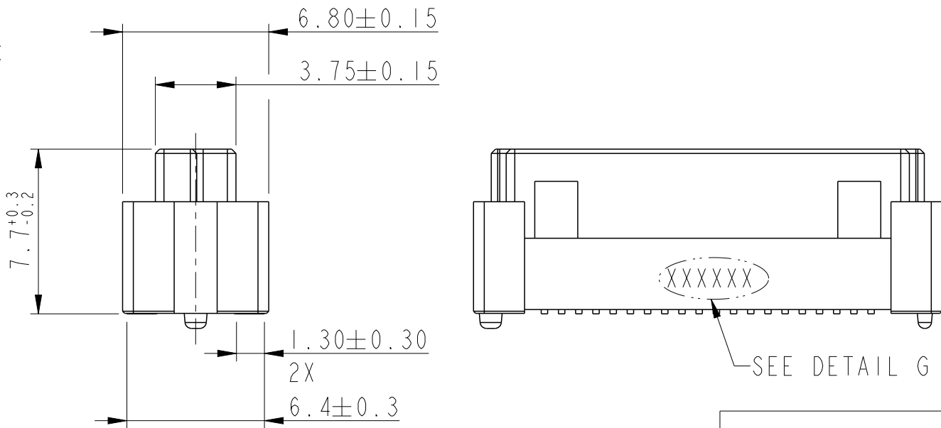
RECEPTACLE 2
