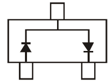
BAT54ST
