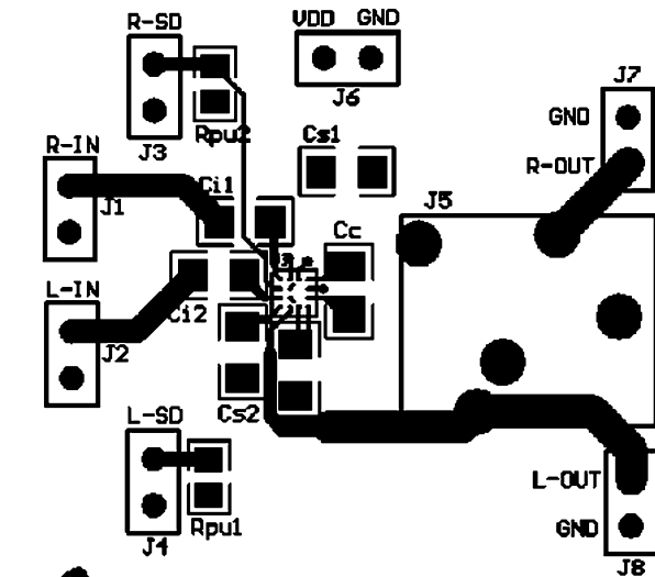
Top Layer
