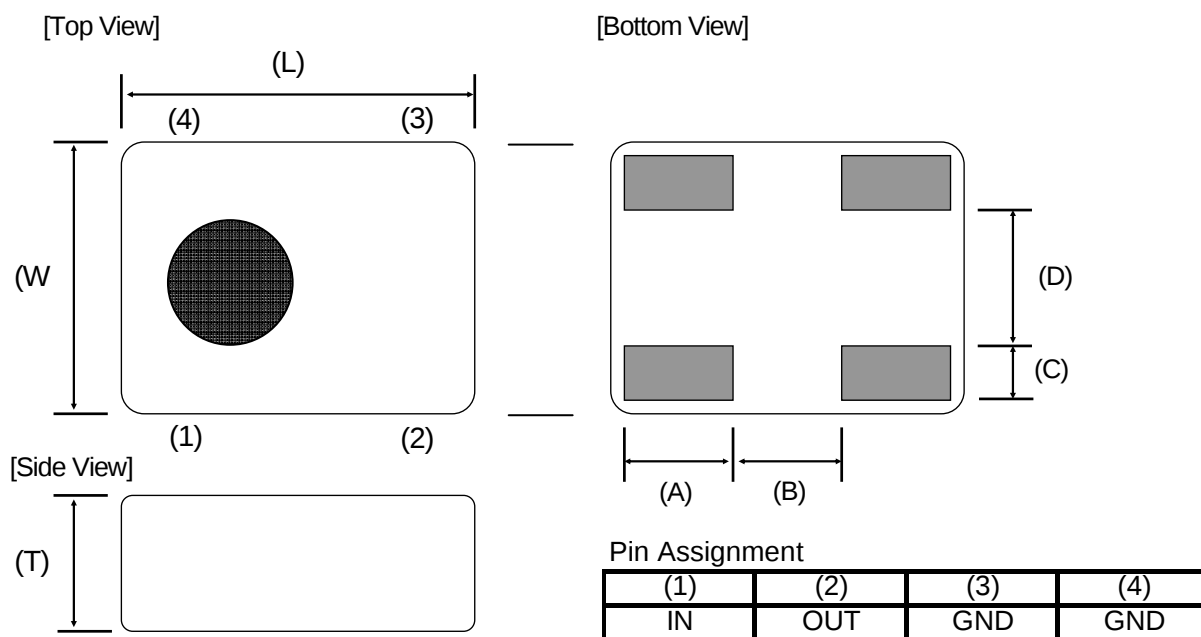
Dimension(mm)
